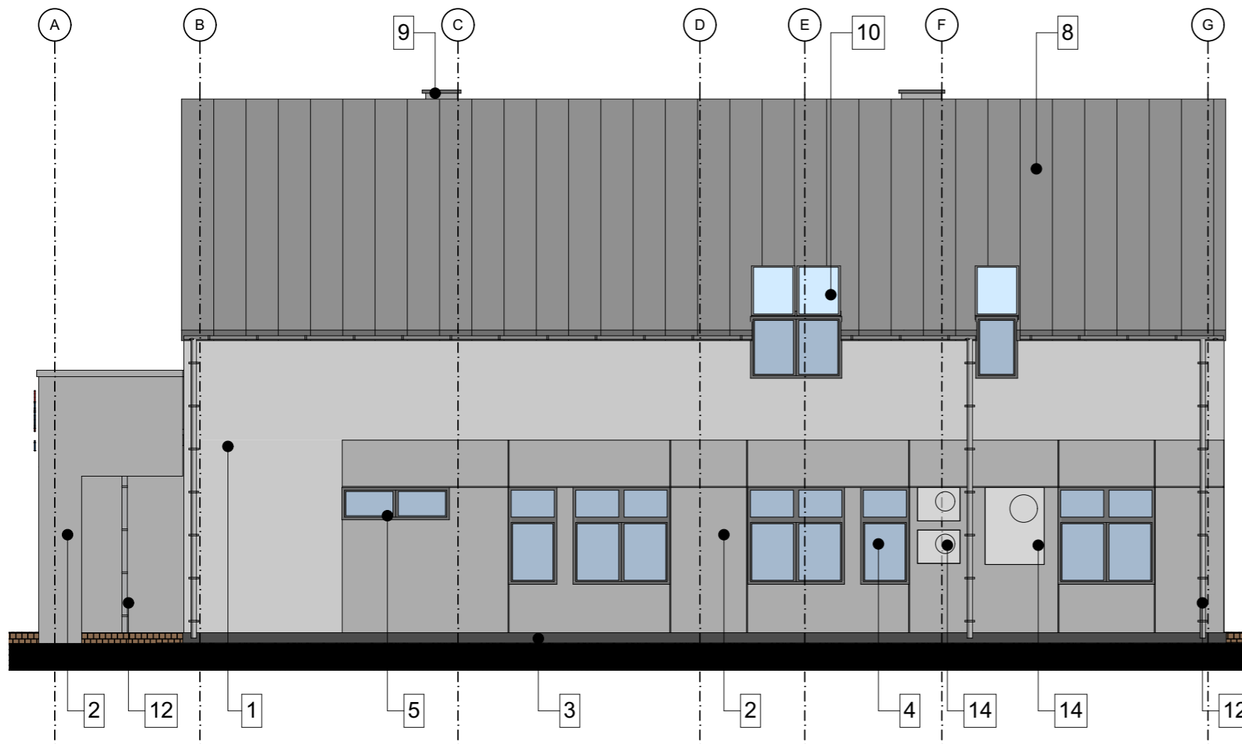
Elewacja Północna
