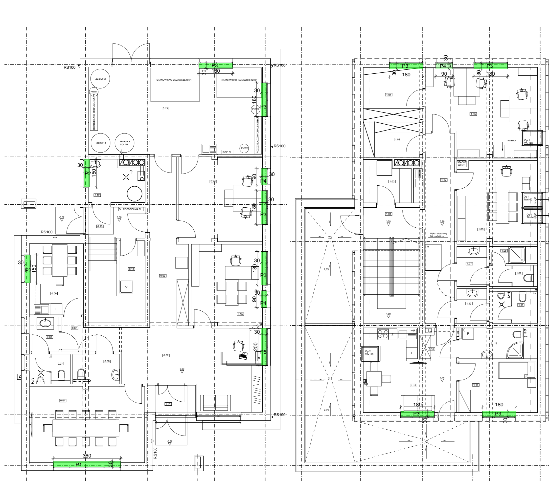
RZUT PARTERU
